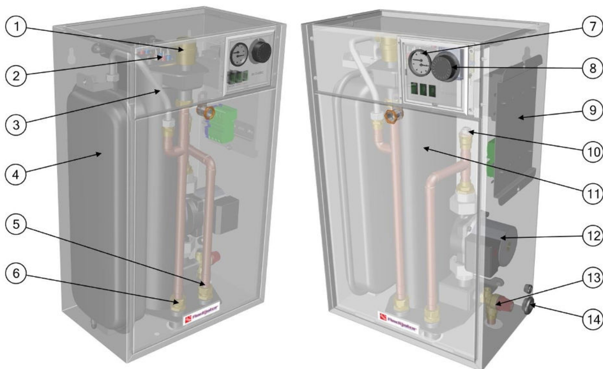
Slika 2. Komponente kotla
