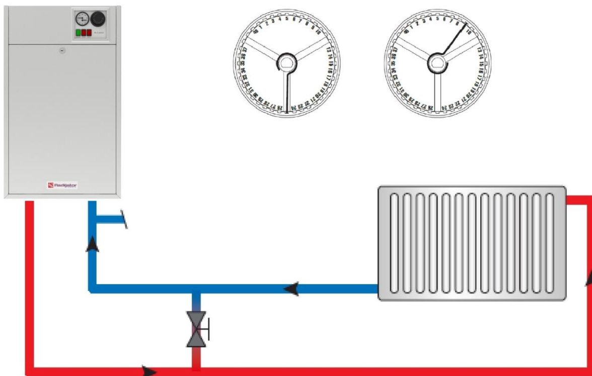
Slika 8. Hidraukička sema centralnog grejanja
