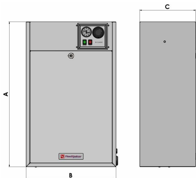
Slika 3. Dimenzije kotla
