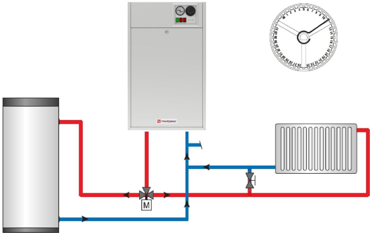
Slika 9. Hidraulička sema „Y“ Plan
