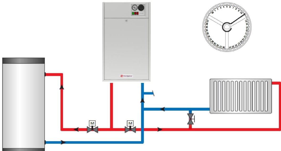
Slika 10. Hidraulička sema "S" Plan
