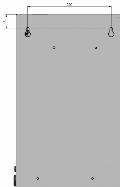
Slika 7. Dimenzije otvora
