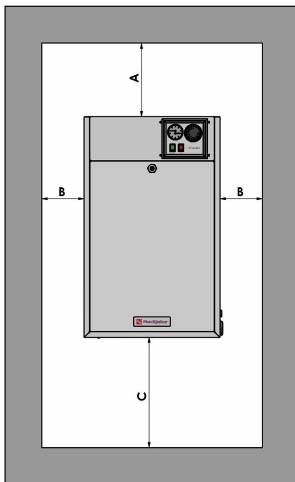
Slika 4. Minimalni razmak nakon montaže kotla
