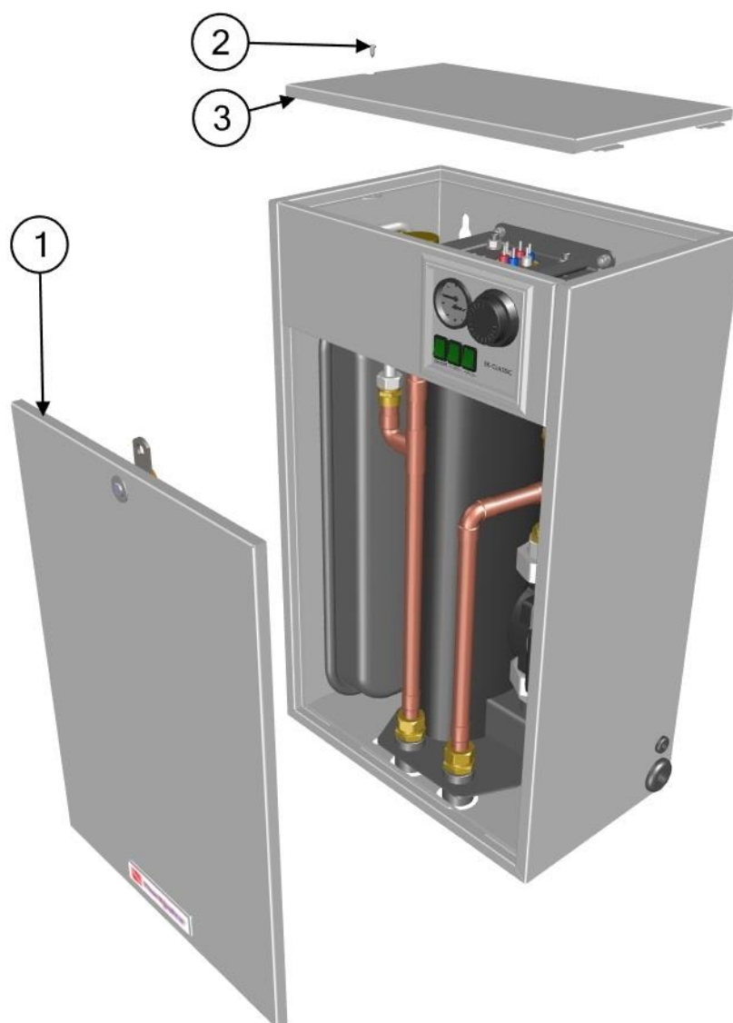
Slika 5. Otvaranje kotla (demontaža prednjeg i gornjeg poklopca kotla)
